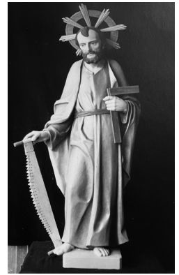
Bilfinger
